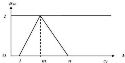
شکل ۳: نمایش عدد فازی مثلثی
